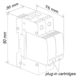
1 Pole
