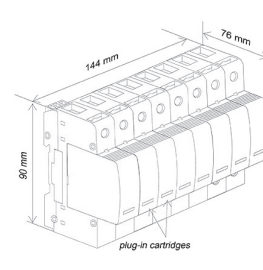
4 Poles
