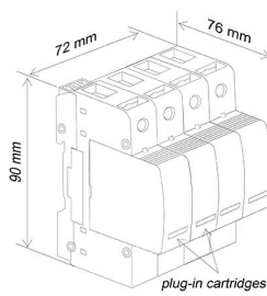
2 Poles
